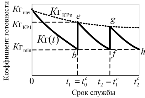
Рис. 10. Расчетная схема динамики коэффициента готовности KГ(t) с проведением КР: KГ_{нач} – начальное значение коэффициента готовности; KГ_{КР1} , KГ_{КРn} – коэффициент готовности машины после первого, n -ного КР; k_{min}^r – значение коэффициента готовности, при котором машина списывается или направляется в КР; t_1, t_2 – моменты времени эксплуатации, в которые машина была направлена в КР; t_0^c, t_1^c, t_2^c – моменты времени, в которые машина должна быть списана соответственно без проведения КР, с проведением одного и двух КР
