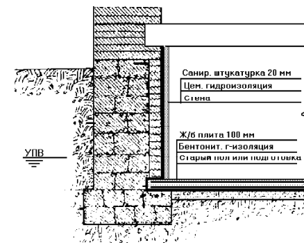
Рис. 20. Гидроизоляция с устройством плиты
