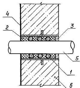
Рис. 14. Пропуск трубопровода через гидроизоляцию с набивным сальником:
