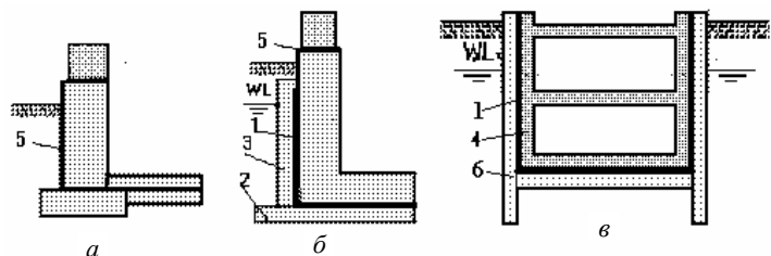
Рис. 16. Устройство гидроизоляции при новом строительстве:
