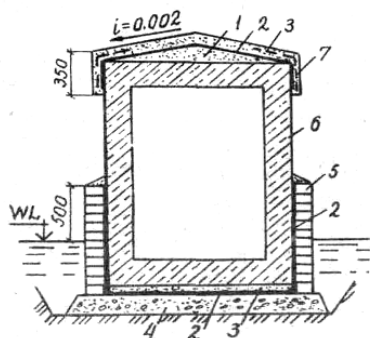
Рис. 10. Комбинированная гидроизоляция:
