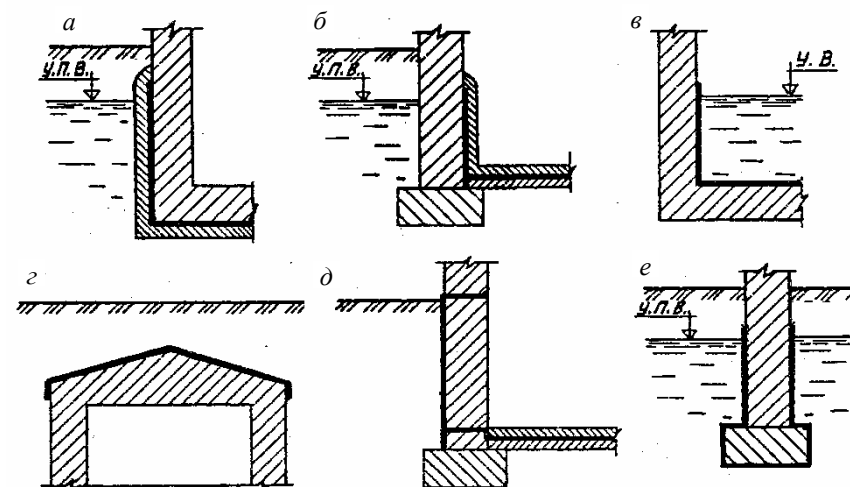
Рис. 6. Виды гидроизоляций для подземных сооружений:
