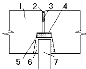
Рис. 9. Межпанельный стык: 1 – наружная стеновая панель; 2 – герметик; 3 – наполнитель; 4 – лента воздухоизоляции самоклеящаяся; 5 – теплоизоляция; 6 – монтажный цементно-песчаный раствор; 7 – внутренняя панель
