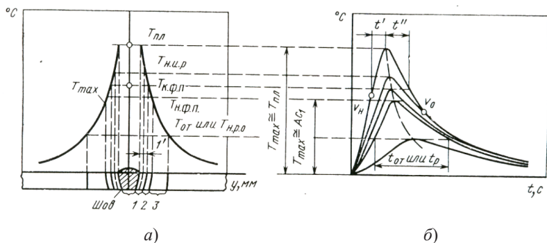
Рис. 43. Строение зон стыкового сварного соединения сталей с полиморфным превращением: а – распределение максимальных температур T_{max} поперек шва и соответствующие им участки зоны термического влияния; б – термические циклы на границах отдельных участков зоны термического влияния: T_{пл} и T_{н.и.р} – температуры плавления и начала интенсивного роста зерна; T_{н.ф.п} и T_{к.ф.п} – температуры начала и конца фазового превращения при нагреве; T_{от} и T_{н.р.о} – температуры отпуска закаленного основного металла перед сваркой и начала рекристаллизации обработки
