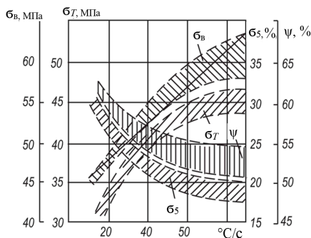
Рис. 46. Зависимость между скоростью охлаждения и механическими свойствами металла шва
