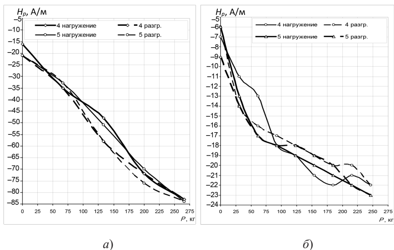
Рис. 50. Зависимость напряженности магнитного поля рассеяния от приложенной нагрузки: а – в зоне с общим коррозионным повреждением; б – в зоне без повреждения
