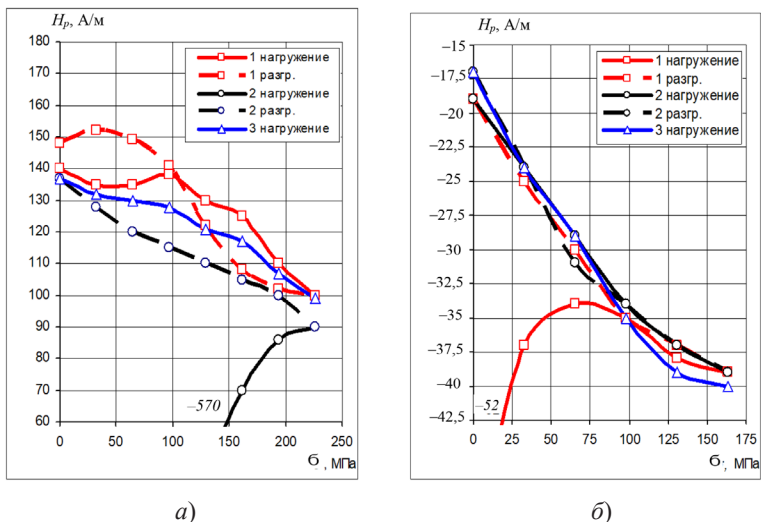
Рис. 16. Зависимость напряженности магнитного поля H_p от одноосных напряжений растяжения \sigma при упругом деформировании намагниченных образцов из стали 08пс (а) и локально упрочненных образцов из стали 10XCHD (б)
