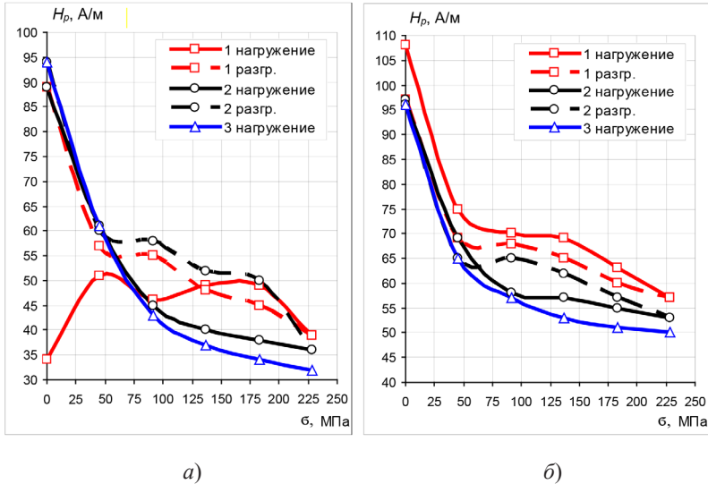
Рис. 42. Зависимость напряженности магнитного поля рассеяния от внутренних напряжений в сварном соединении из стали Ст3 со снятым усилением: а – в зоне сплавления основного металла со сварным швом; б – в зоне основного металла
