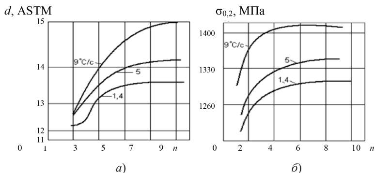
Рис. 17. Влияние числа циклов n и скорости нагрева на размер зерна d аустенита (а) и условный предел текучести \sigma_{0.2} стали, содержащей 5 % Ni (б)
