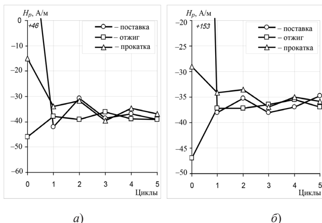
Рис. 19. Зависимость напряженности магнитного поля H_p от числа циклов при термоциклировании сталей 08пс (а) и 10XСНД (б) в различных исходных структурных состояниях
