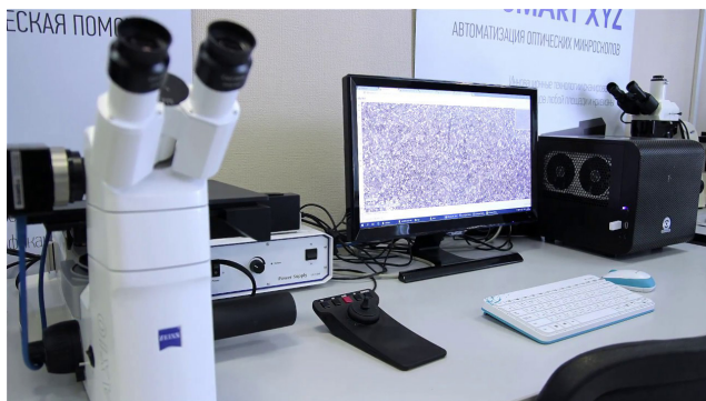
Рис. 14. Комплекс приборов для проведения металлографического анализа
