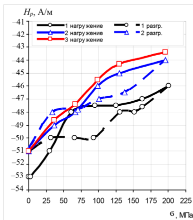
Рис. 32. Зависимость напряженности магнитного поля H_p от относительных напряжений сжатия \sigma образцов из сталей Ст3 в состоянии поставки
