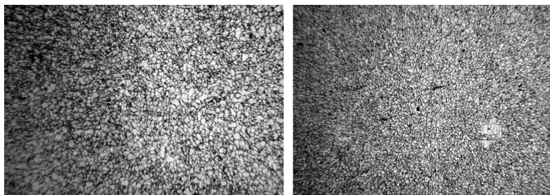
Рис. 27. Изменение структуры стали 10XСНД при термоциклической обработке, \times 650 : а – состояние «поставка + прокатка на \epsilon = 50\% »; б–е – после 1–5-го циклов соответственно
