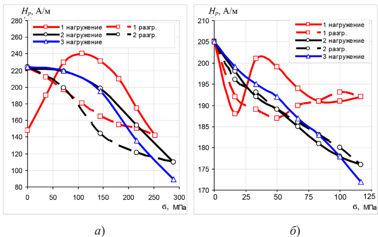
Рис. 28. Зависимость напряженности магнитного поля рассеяния H_p от одноосных напряжений растяжения \sigma образцов из сталей в состоянии поставки: а – 10XСНД; б – 08пс
