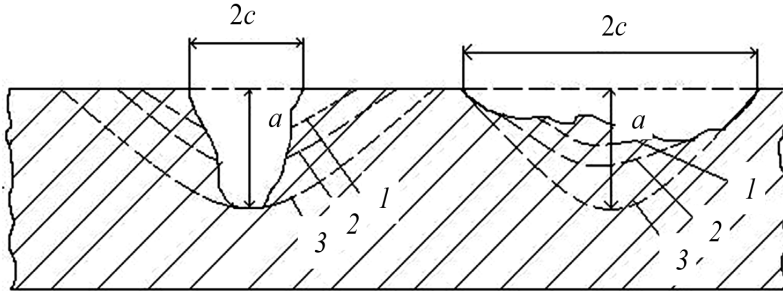
Рис. 9. Развитие поверхностных трещин в коррозионных концентраторах
