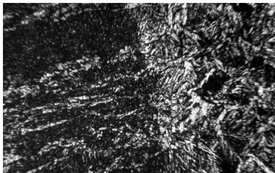
Рис. 44. Микроструктура стыкового сварного соединения из стали Ст3 в зоне сварного шва и зоне сплавления, \times 200
