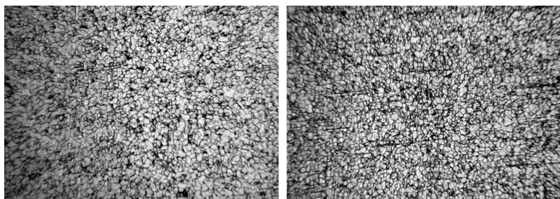
Рис. 23. Изменение структуры стали 08пс при термоциклической обработке, \times 650 : а – состояние «поставка + отжиг при 900\text{ }^{\circ}\text{C} »; б–е – после 1–5-го циклов соответственно
