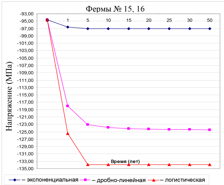
Рис. 59. Изменение расчетных внутренних напряжений в элементах крупномасштабной сварной фермы № 15, 16 при эксплуатации в условиях воздействия коррозионной среды
