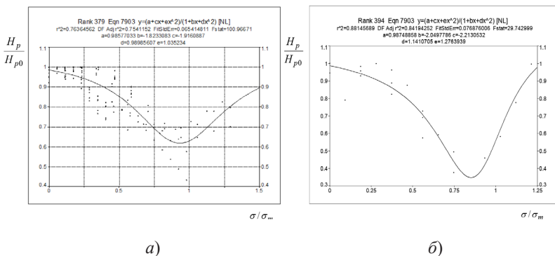
Рис. 40. Графическое представление регрессионных зависимостей для стали 10XСНД: а – частная зависимость (состояние поставки); б – обобщенная (совокупность структурных состояний)
