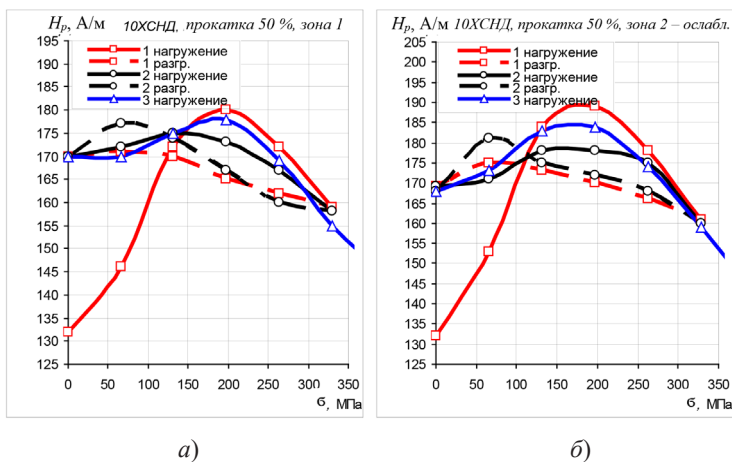
Рис. 31. Зависимость напряженности магнитного поля H_p от одноосных напряжений при упругом растяжении образцов из стали 10ХСНД, подвергнутых предварительной прокатке на \epsilon = 50\% : a – с неослабленным (зона 1) сечением; б – с ослабленным (зона 2) сечением
