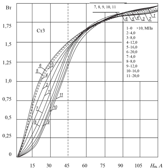
Рис. 11. Изменение кривой намагничивания стали Ст3 под действием нагрузки
