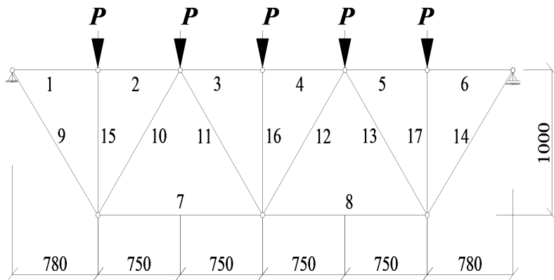
Рис. 52. Схема нагружения крупномасштабной модели сварной фермы
