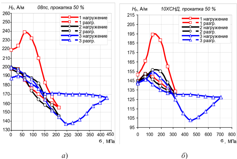
Рис. 37. Зависимость напряженности магнитного поля H_p от одноосных напряжений растяжения для образцов из сталей в состоянии поставки + прокатки на \varepsilon = 50\% : а – 08пс; б – 10ХСНД
