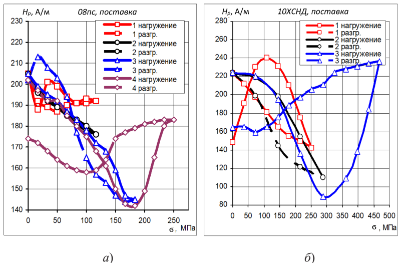
Рис. 35. Зависимость напряженности магнитного поля H_p от одноосных напряжений растяжения для образцов из сталей в состоянии поставки: а – 08пс; б – 10ХСНД
