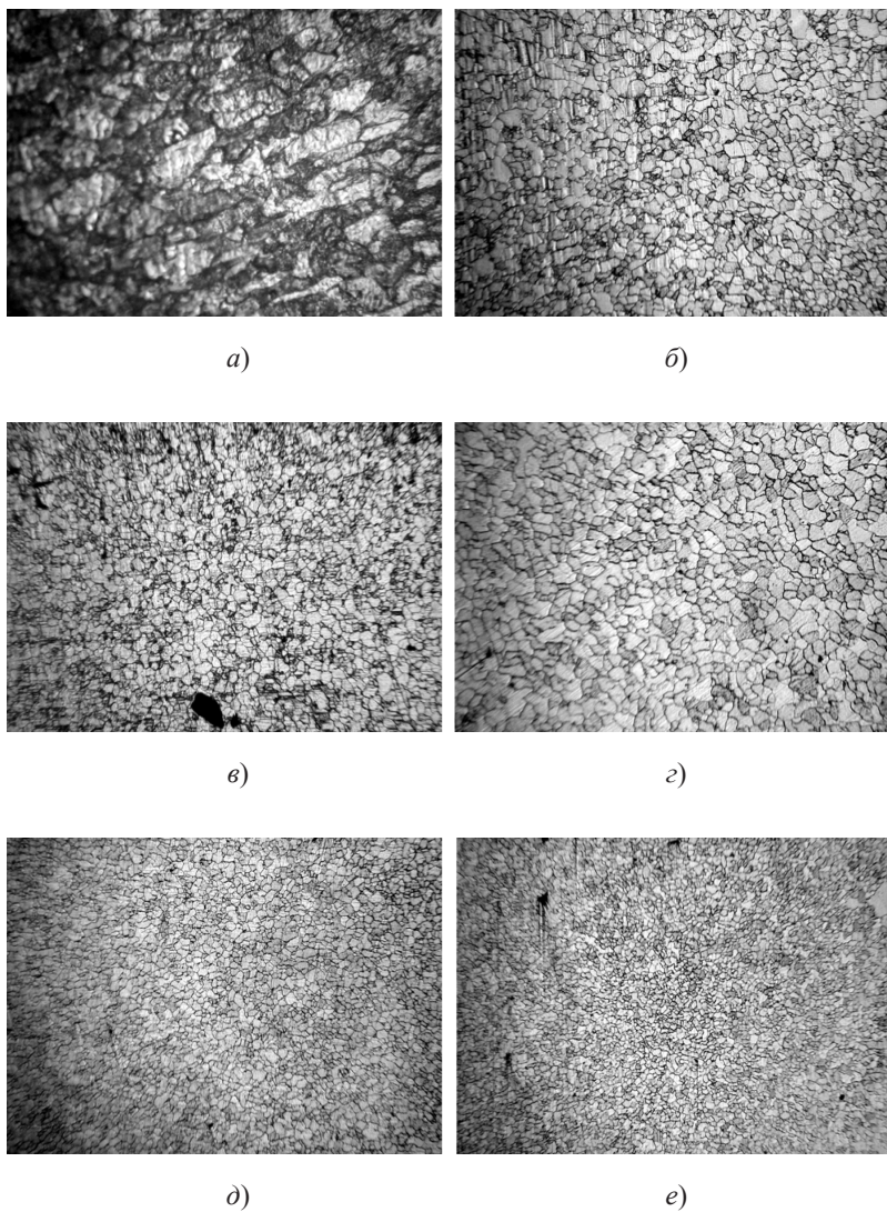
Рис. 24. Изменение структуры стали 08пс при термоциклической обработке, \times 650 : a – состояние «поставка + прокатка на \epsilon = 50\% »; б–е – после 1–5-го циклов соответственно
