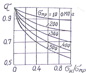
Рис. 3. Зависимость относительной долговечности стали от различных уровней прочности
