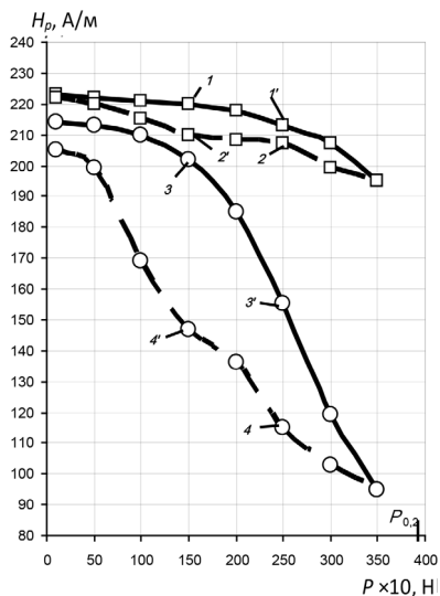
Рис. 49. Зависимость напряженности магнитного поля рассеяния H_p от приложенной нагрузки в зонах 1 (с локальным коррозионным повреждением) и 2 (без повреждения)
