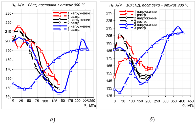
Рис. 34. Зависимость напряженности магнитного поля H_p от одноосных напряжений растяжения для образцов из сталей в состоянии поставки + отжига при 900 °С: а – 08пс; б – 10ХСНД
