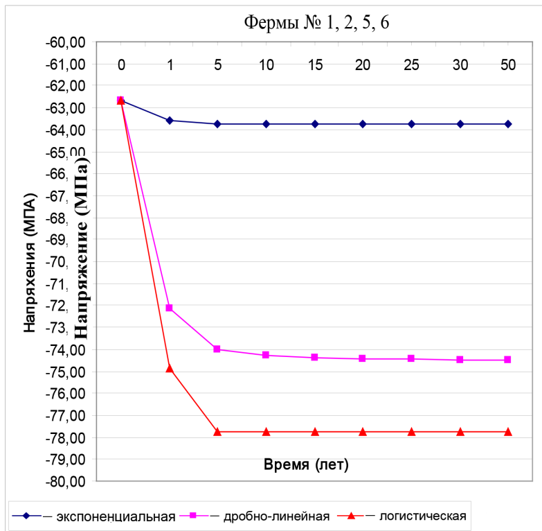
Рис. 53. Изменение расчетных внутренних напряжений в элементах крупномасштабной сварной фермы № 1, 2, 5, 6 при эксплуатации в условиях воздействия коррозионной среды
