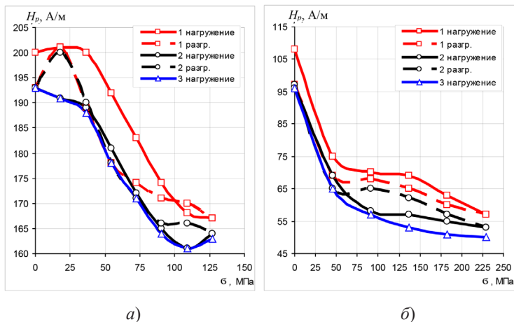
Рис. 30. Зависимость напряженности магнитного поля H_p от одноосных напряжений растяжения \sigma образцов из сталей: a – 08пс после отжига при 900 °С; б – СтЗ в состоянии поставки
