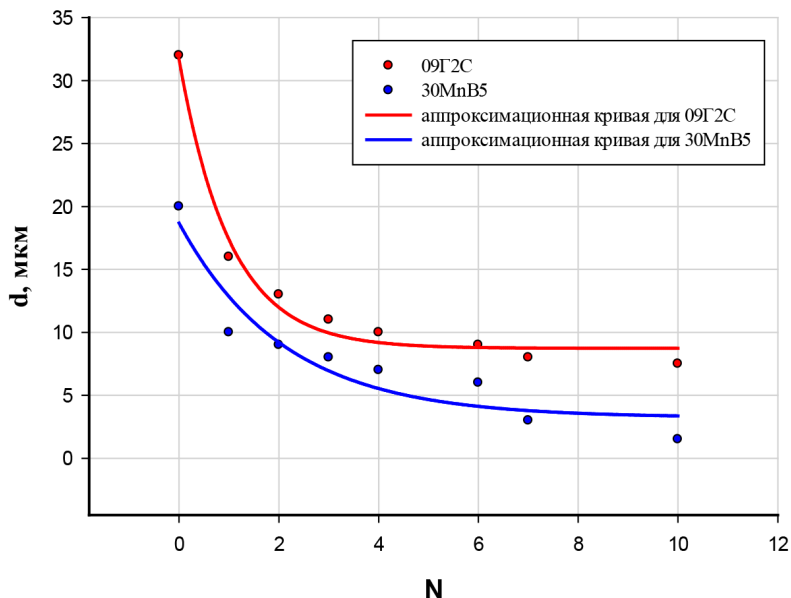
Рис. 63. Зависимость d = f(N)
