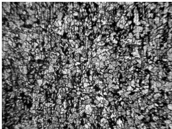
Рис. 48. Микроструктура стыкового сварного соединения из стали Ст3 в зоне основного металла
