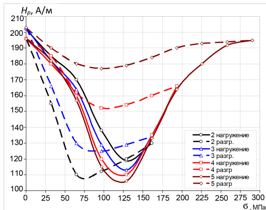
Рис. 39. Зависимость напряженности магнитного поля рассеяния H_p от одноосных напряжений растяжения \sigma при циклическом нагружении и разгрузке образцов из стали 08кп (состояние поставки) в области пластического деформирования
