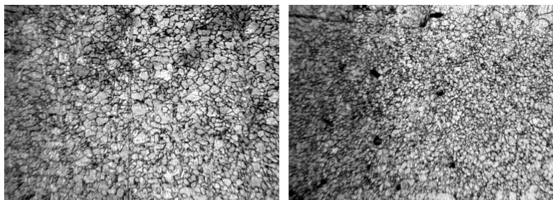
Рис. 25. Изменение структуры стали 10ХСНД при термоциклической обработке, \times 650 : а – состояние поставки; б–е – после 1–5-го циклов соответственно
