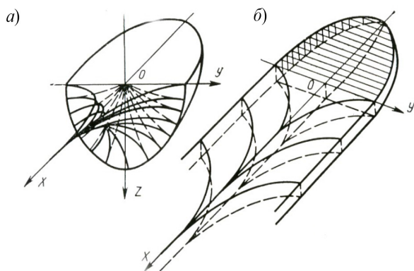
Рис. 45. Траектории роста кристаллитов в сварочной ванне при схемах кристаллизации: a – пространственной; б – плоской
