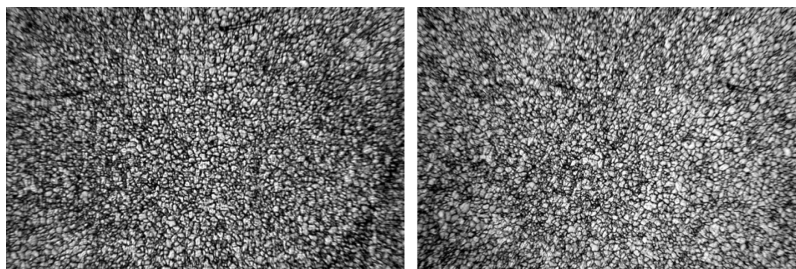
Рис. 22. Изменение структуры стали 08пс при термоциклической обработке, \times 650 : а – состояние поставки; б–е – после 1–5-го циклов соответственно
