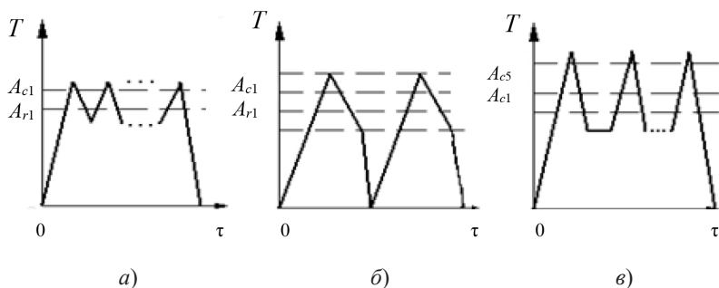
Рис. 18. Схемы ТЦО сталей:
