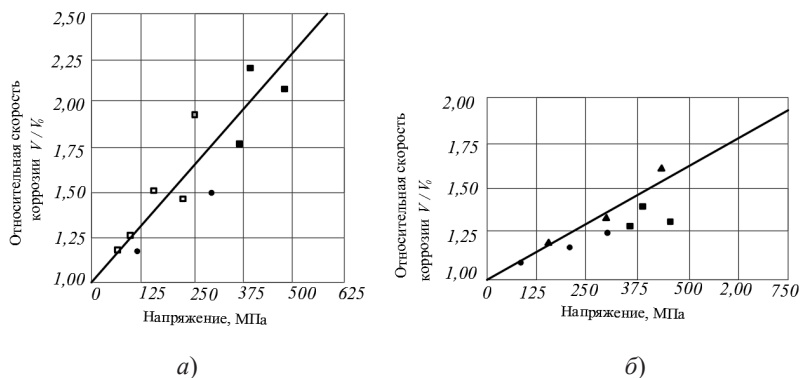
Рис. 1. Относительная скорость коррозии сталей ( \square – Ст3, \bullet – сталь 20, \blacksquare – сталь 45, \blacktriangle – сталь У8) в зависимости от схемы напряженно-деформированного состояния: а – плоское; б – одноосное
