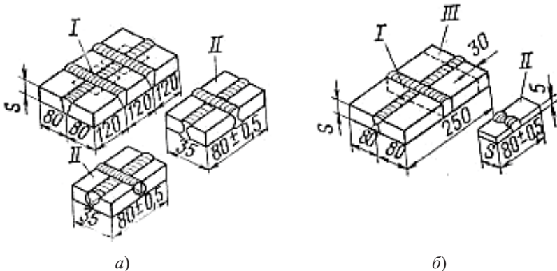
Рис. 7. Образцы для испытания на межкристаллитную коррозию: а – при толщине металла до 10 мм; б – при толщине металла более 10 мм; I – место вырезки образца; II – контрольная поверхность; III – отход; S – толщина металла
