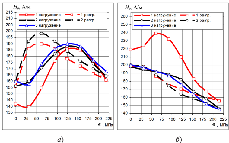
Рис. 29. Зависимость напряженности магнитного поля H_p от одноосных напряжений растяжения \sigma образцов из сталей: а – 10XСНД в состоянии поставки + ТЦО; б – 08пс после прокатки на \epsilon = 50\%
