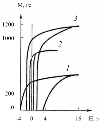
Рис. 38. Влияние вида обработки на форму петли магнитного гистерезиса: 1 – после наклепа; 2 – после отжига; 3 – кривая мягкого железа (для сравнения)
