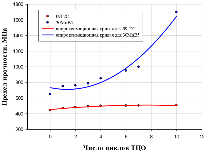
Рис. 64. Зависимости \sigma_{0,2} = f(N) и \sigma_b = f(N)
