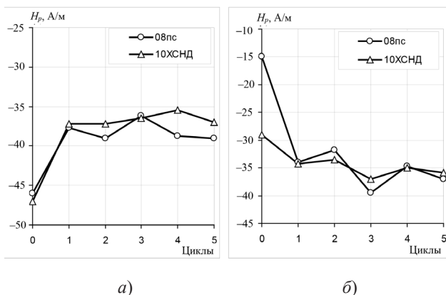
Рис. 21. Зависимость напряженности магнитного поля рассеяния H_p от числа циклов при термоциклировании сталей 08пс и 10ХСНД после предварительного отжига при 900 °С (а) и холодной пластической деформации на \epsilon = 50\% (б)
