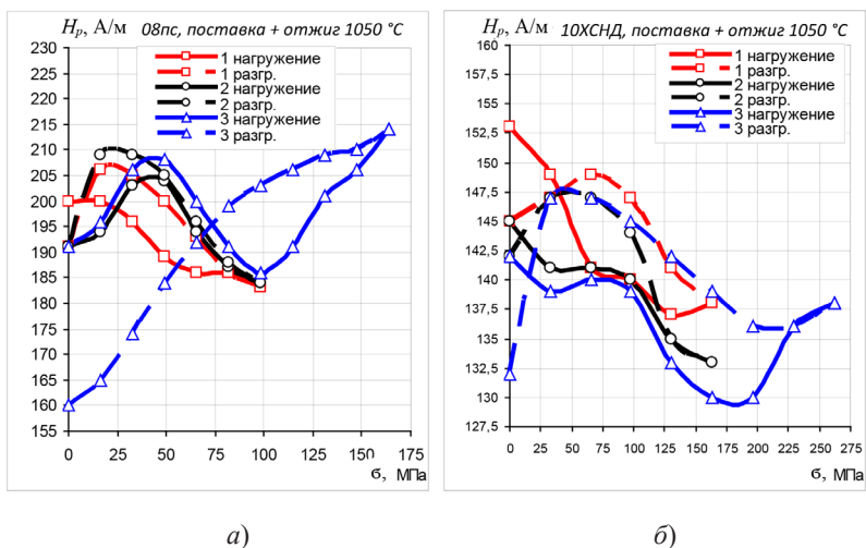
Рис. 33. Зависимость напряженности магнитного поля H_p от одноосных напряжений растяжения для образцов из сталей в состоянии поставки + отжига при 1050 °С: а – 08пс; б – 10ХСНД
