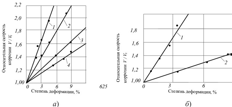
Рис. 2. Зависимость относительной скорости коррозии V_{\varepsilon} / V_0 образцов от степени деформации \varepsilon : а – графики: 1 – сталь 45 (закалка + отпуск, V_0 = 0,0084 мм/ч); 2 – сталь Ст3 ( V_0 = 0,01 мм/ч); 3 – сталь 45 (нормализация, V_0 = 0,0075 мм/ч); 4 – сталь 20 ( V_0 = 0,0118 мм/ч); б – графики: 1 – сталь 16Г (закалка + отпуск); 2 – сталь 16Г (нормализация)
