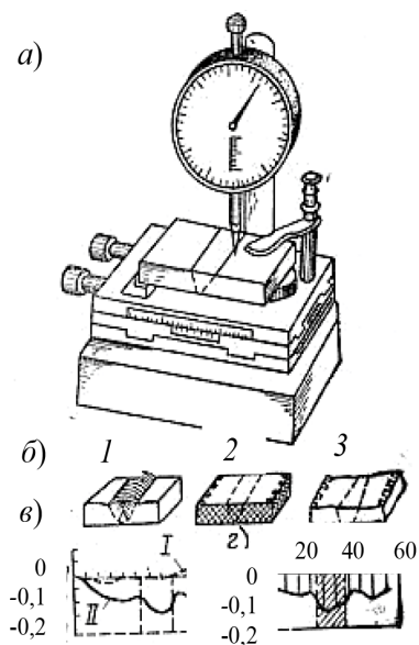
Рис. 5. Испытания на коррозионную стойкость шва профилометром:
